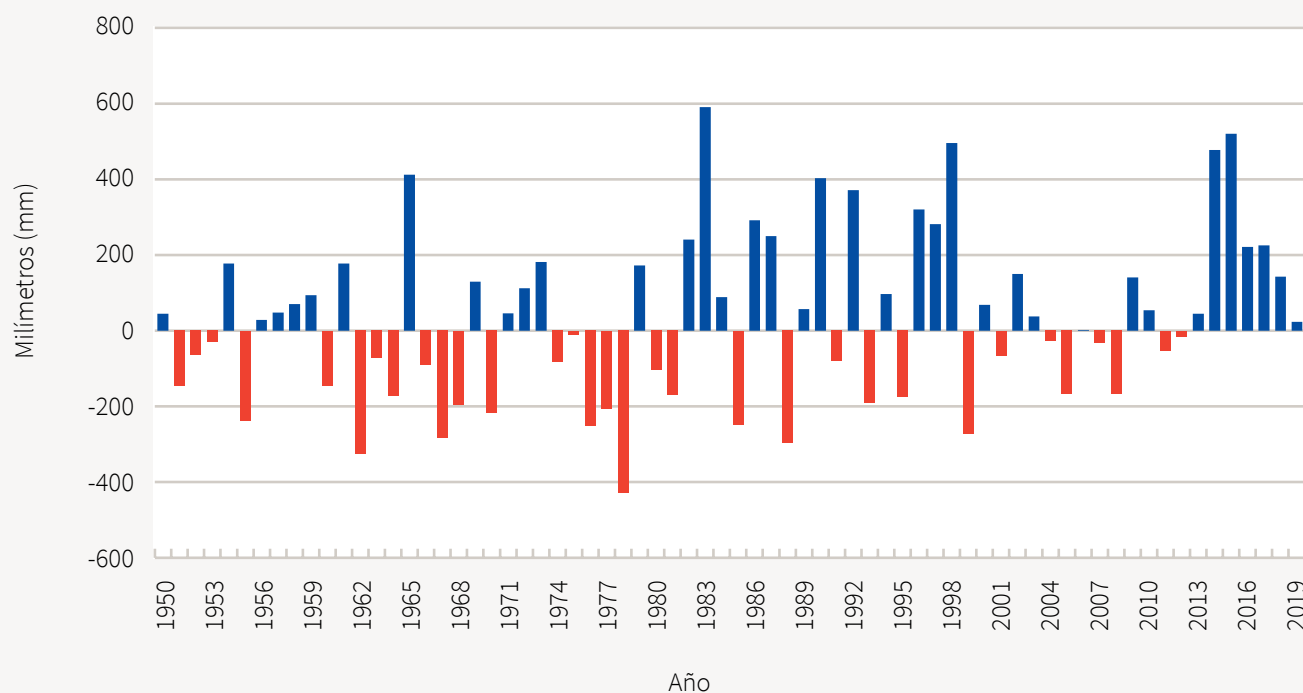
Gráfico 13. Anomalía de la precipitación total media anual en Paraguay durante 1950-2019 respecto de la precipitación total normal del periodo 1961-1990 (1464 mm). Barra azul exceso y barra roja déficit.
