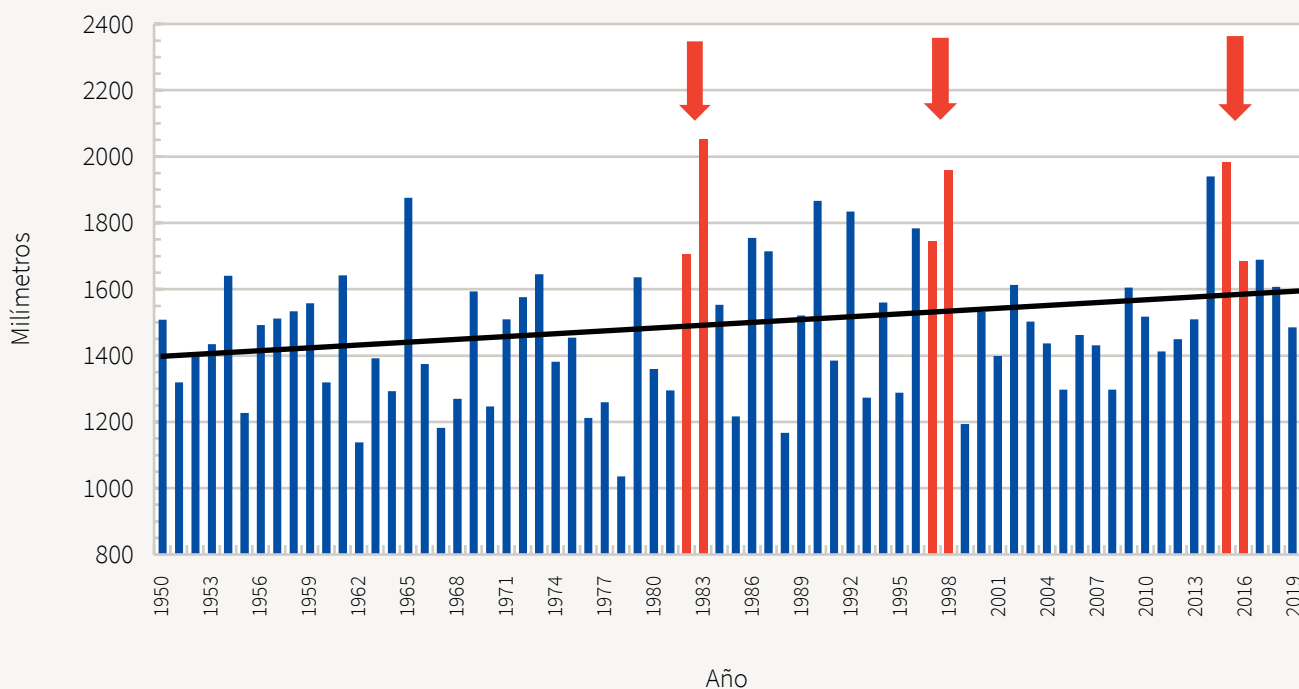
Gráfico 12. Precipitación total media anual en el Paraguay (barra azul) y tendencia lineal (línea negra). Flecha vertical indica años con El Niño fuerte ( \Delta TSM \geq 1,5^\circ C ) 50 . Período 1950-2019.
