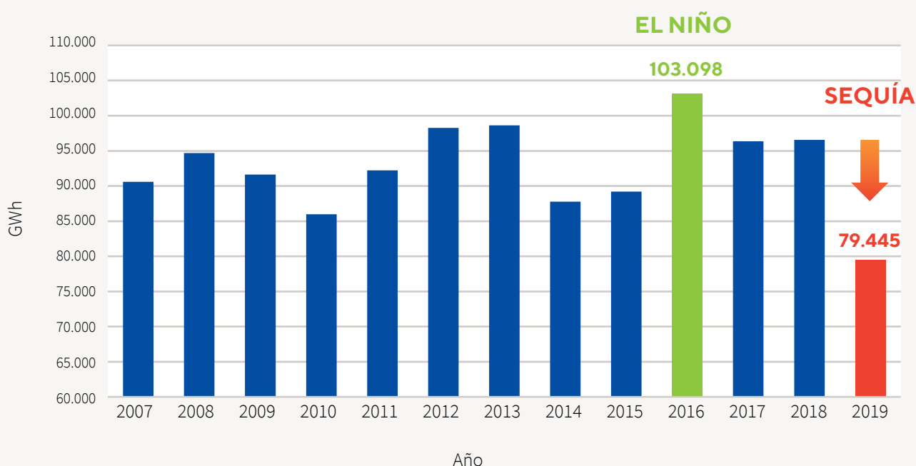
Gráfico 27. Producción anual de energía eléctrica en IB con 20 unidades generadoras en el período 2007-2019. Producción máxima en el año 2016 por efecto de El Niño 2015-2016 (barra verde) y producción mínima por efecto de la sequía del año 2019 (barra roja).
