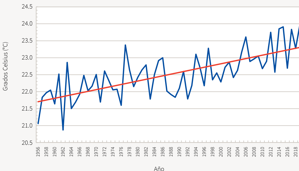
Gráfico 2. Temperatura media anual en Villarrica, Guairá (promedio de temperaturas máximas y mínimas diarias). Periodo 1956-2019.
