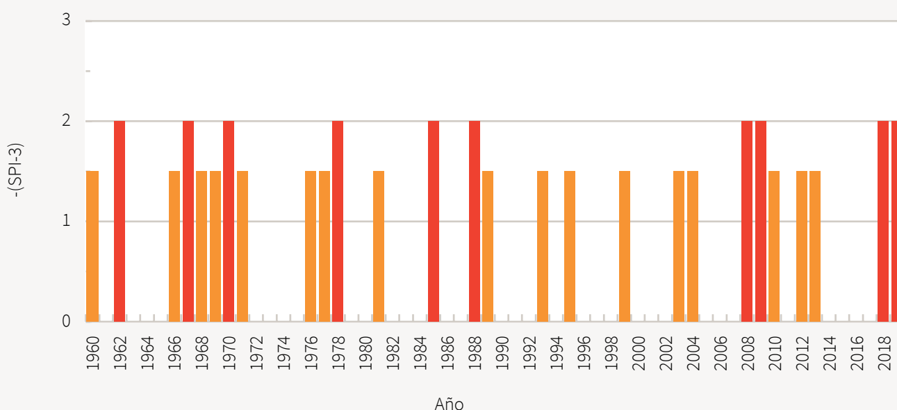
Gráfico 21. Años con sequías moderadas (barra color ocre) y sequías fuertes (barra color marrón) en Paraguay en el período 1960-2019. Escala vertical solo valores de SPI-3 negativos. Estos casos consideran sequías que han cubierto al menos una gran parte del territorio.
